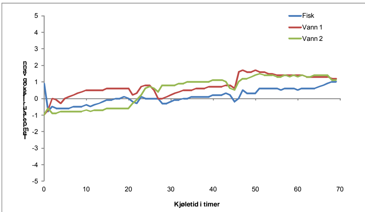
Figur 4 Temperaturlogg fra CSW forsøket med høy vanntemperatur .
